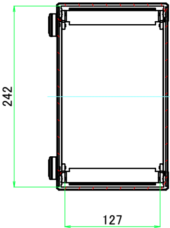
B-B ( 1 : 5 )
