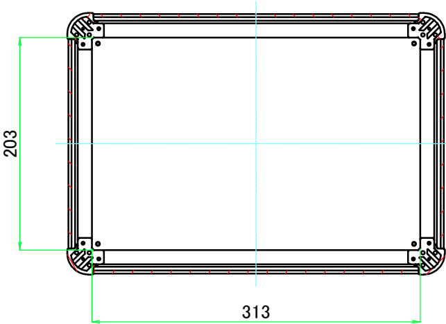
C-C ( 1 : 5 )
